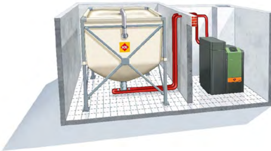
Schema einer Holzpelletheizung mit Sacksilo (Quelle: HDG-Bavaria GmbH, Massing)
