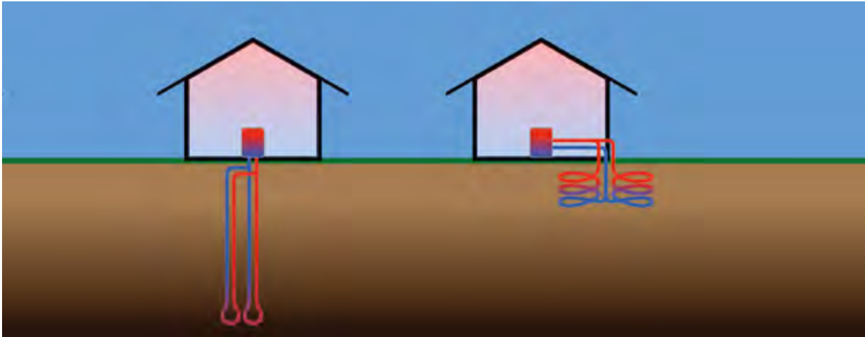
Beispiel: Geothermie-Systeme (Wärmepumpe mit Erderwärmesonde (Tiefenbohrung) bzw. Erdkollektoren)
