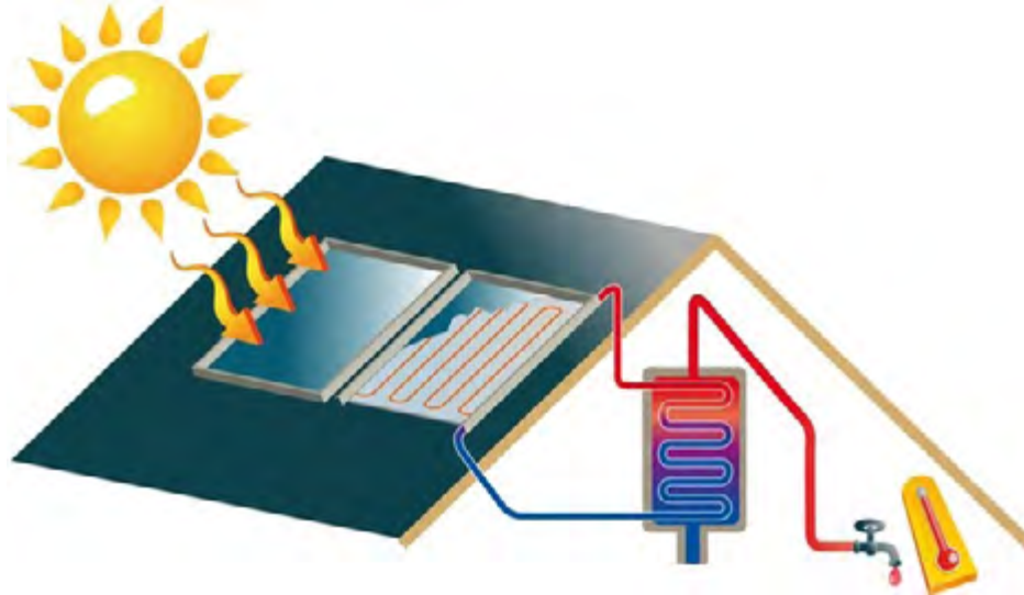
System zur solarthermischen Warmwassererzeugung (Quelle: Solarthermie.net)
